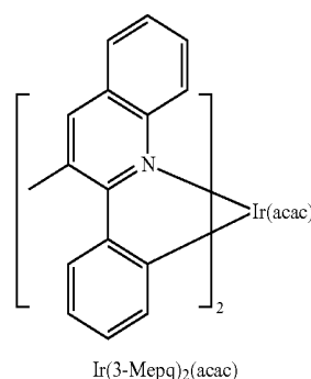
Ir(3-Mepq) 2 (acac)
