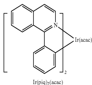
Ir(piq) 2 (acac)
